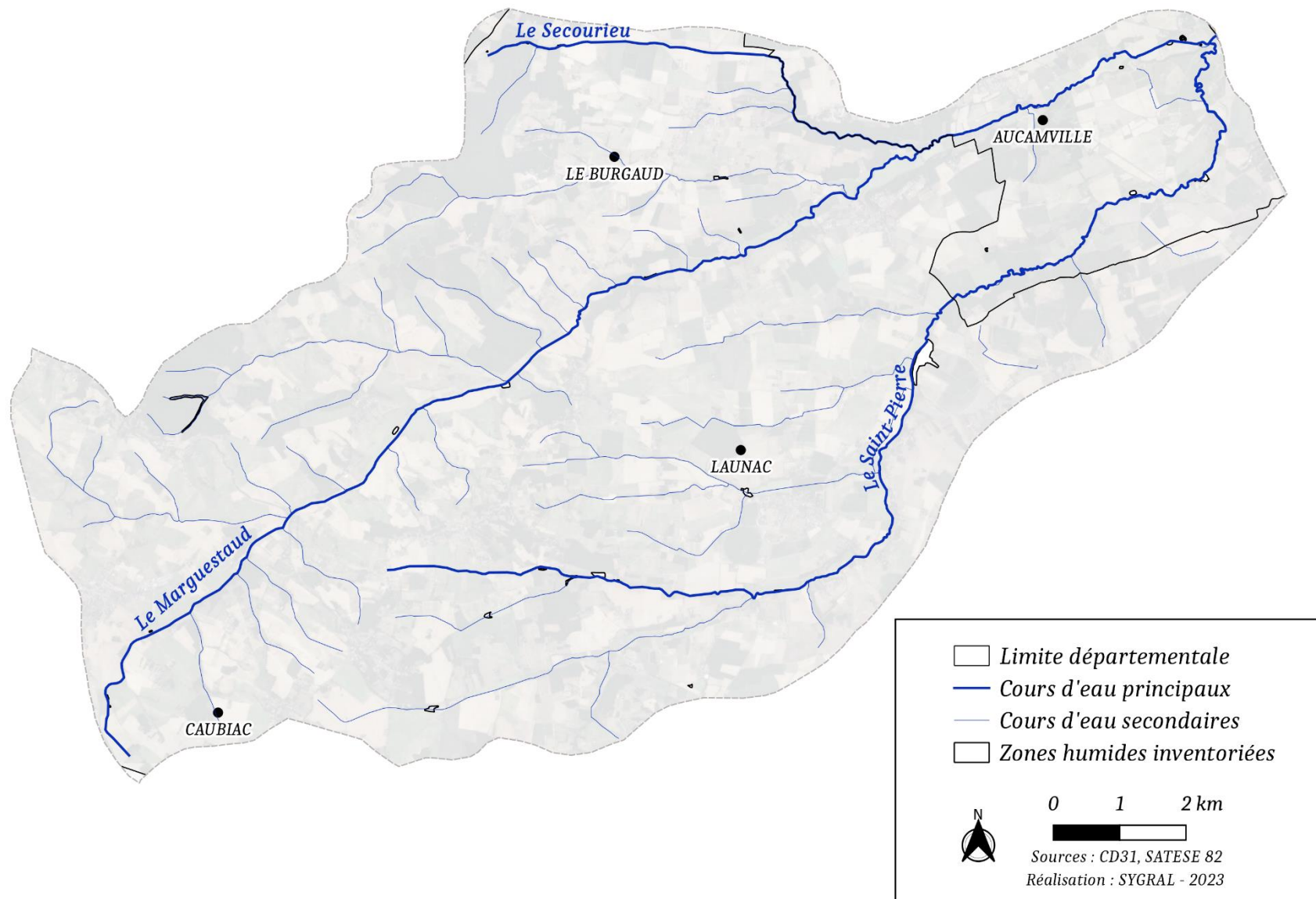
Annexe 9.d – Cartographie des zones humides recensées sur le bassin versant du Marguestaud
